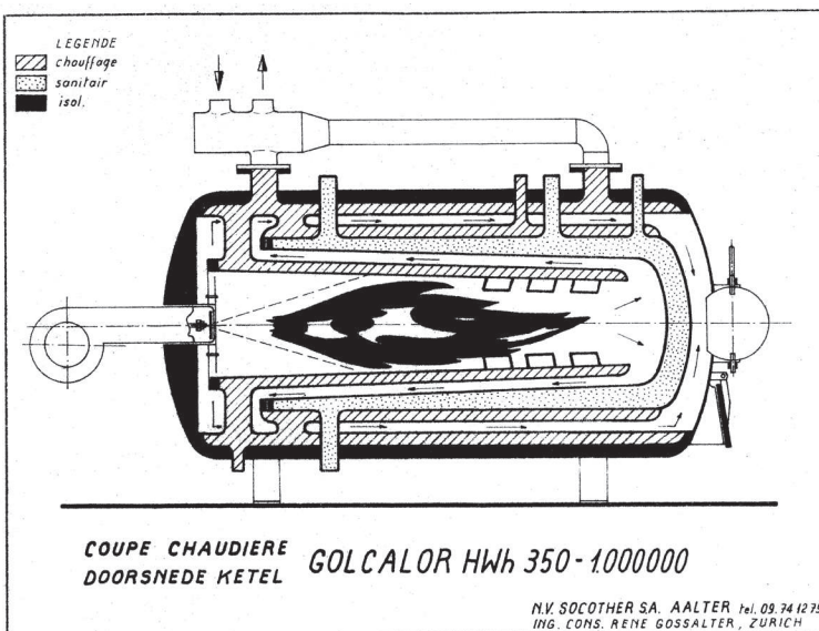
Een doorsnede van het eerste model golcalorketel volgens een ontwerp van Gossalter dat getekend werd door Gisèle Hooft.
