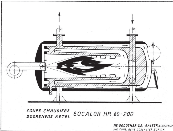
Een doorsnede van het eerste model socalorketel volgens een ontwerp van Gossalter dat getekend werd door Gisèle Hooft.
