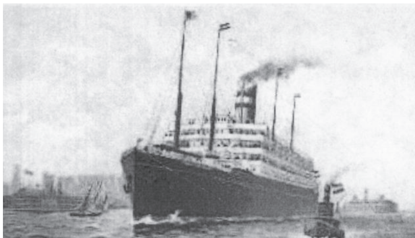
Nieuw-Amsterdam. In 1906 te Belfast gebouwd door Harland & Wolff voor de Holland-Amerika Line; lengte 600,3 feet en breedte 68,9 feet.
