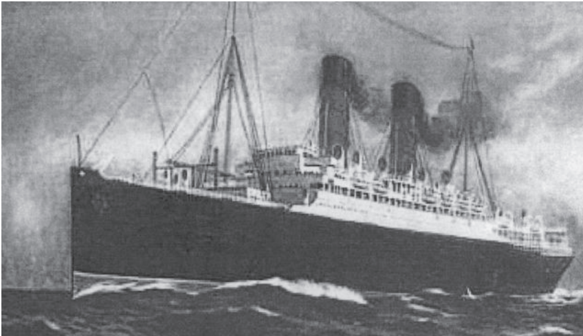
RMS Franconia. Gebouwd te Wallesend-on-Tyne door Wigham Richardson in England voor de Cunard Line. Gelanceerd in juli 1910; maidentrip februari 1911. Liverpool-Queensland-New York. In 1915 troepen- transportschip; getorpedeerd door Duitse U 47 bij Malta; 18 150 bruto ton; afmetingen: lengte 600 feet, breedte 71,3 feet.
