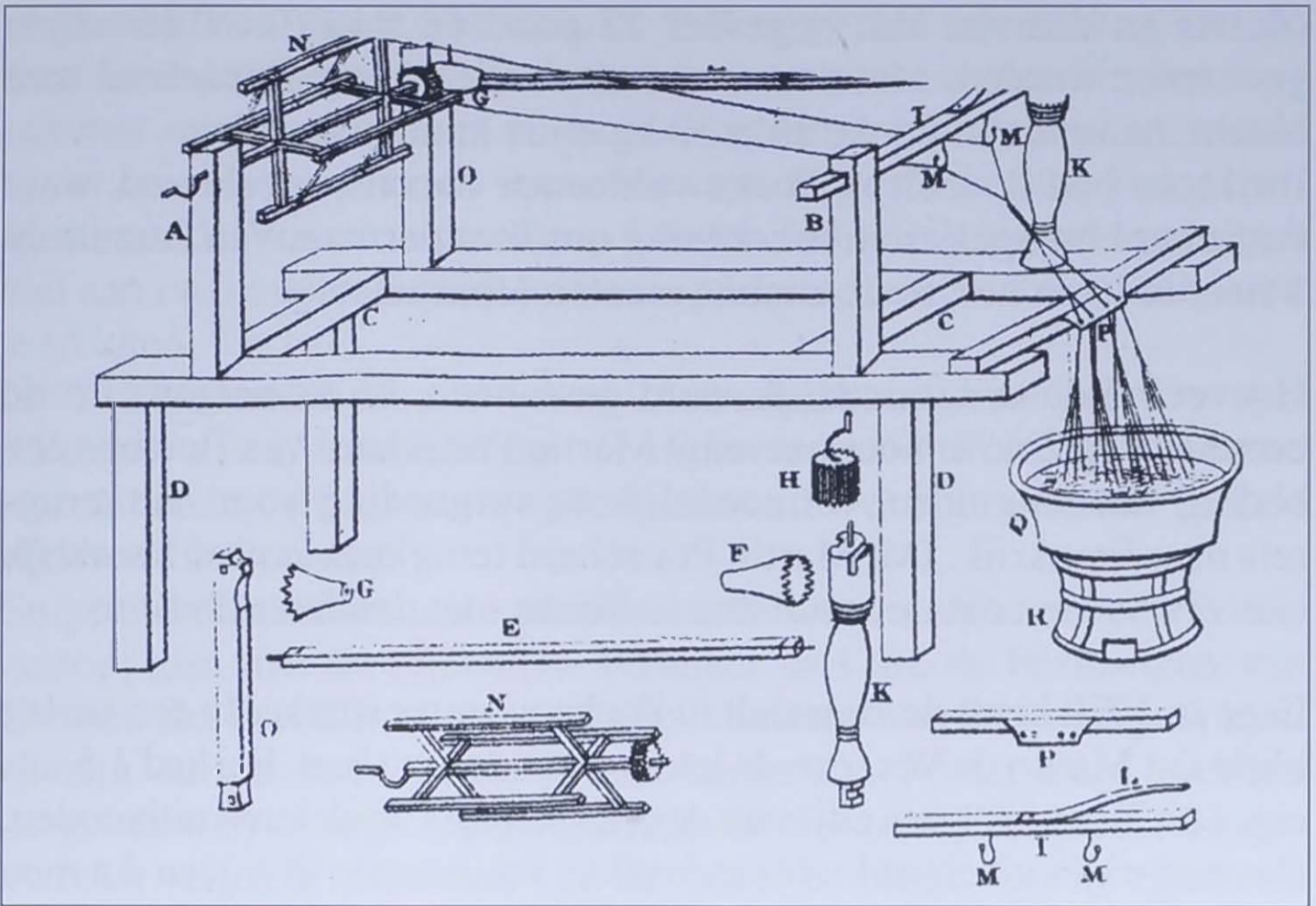
Installatie om de cocons af te haspelen en zijdedraad te spinnen. Naar Vincenzo Dandolo. (32)
