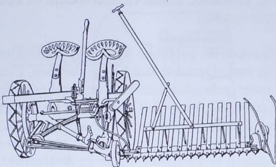
Eenvoudige pikmachine getrokken door een paard. Een begeleider verzamelt het koren met een rakel tot schoven. (4)
