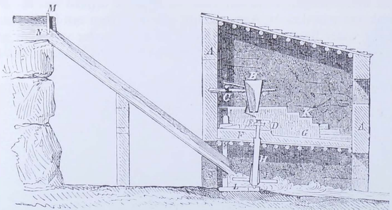
Schematische voorstelling van een Arabische watermolen. Naar: Baumgarten F. (14)
