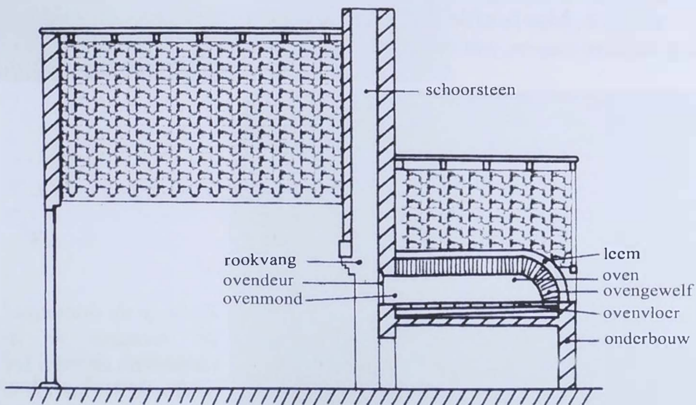
Tekening die de doorsnede van een bakhuis weergeeft. Naar: Johan van Twembeke.
