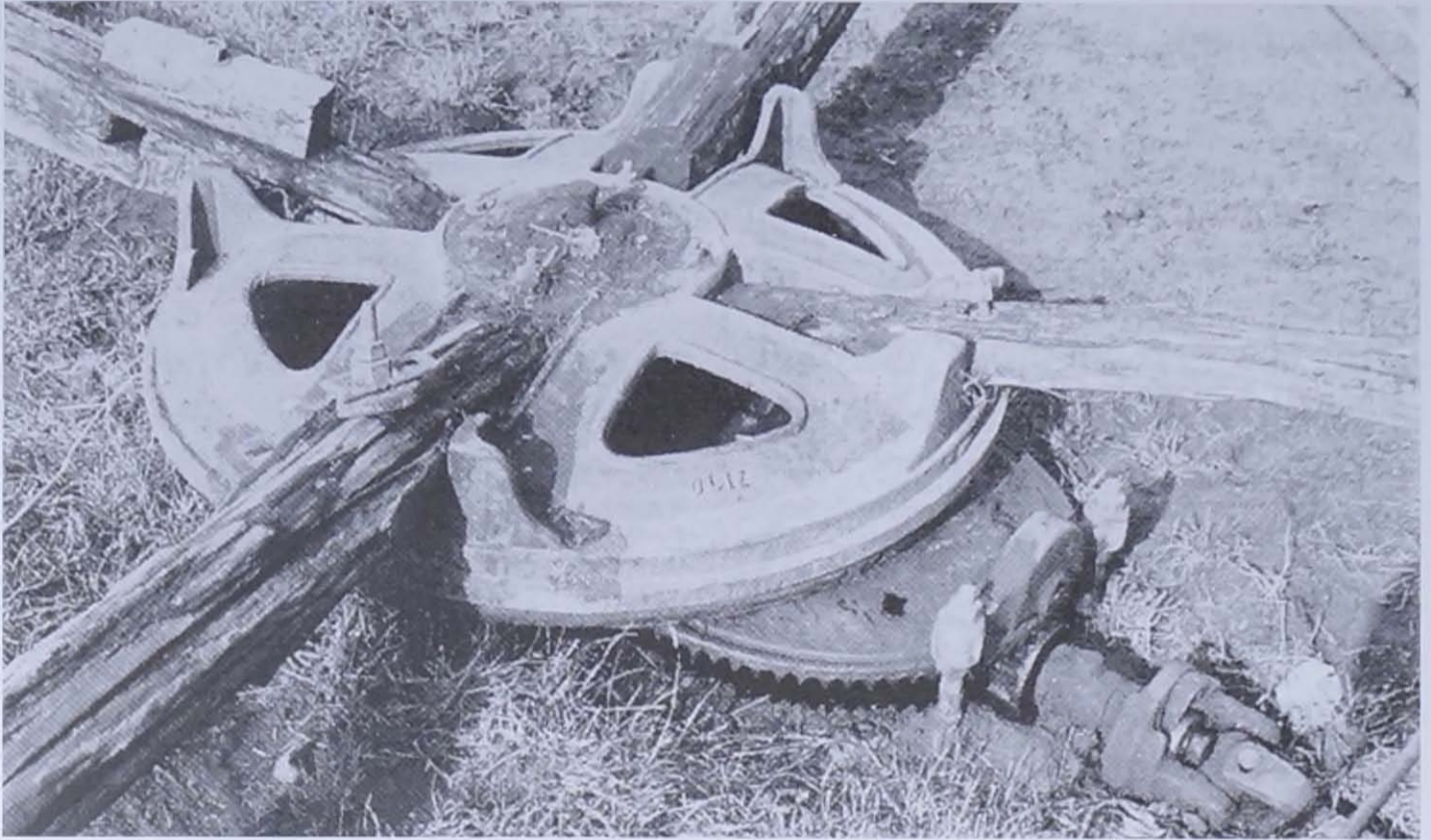
Aandrijfmechanisme van een paardenmanege. (13)
