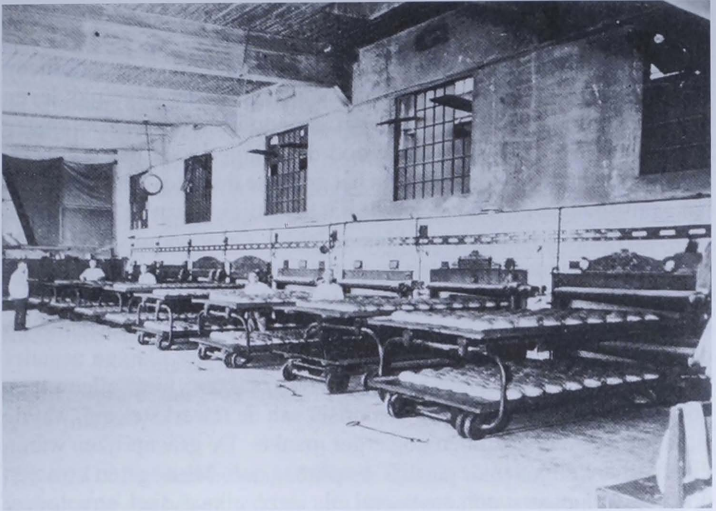
Uitrolbare heetwaterovens in de Coöperatieve Vooruit in Gent anno 1914. (33)
