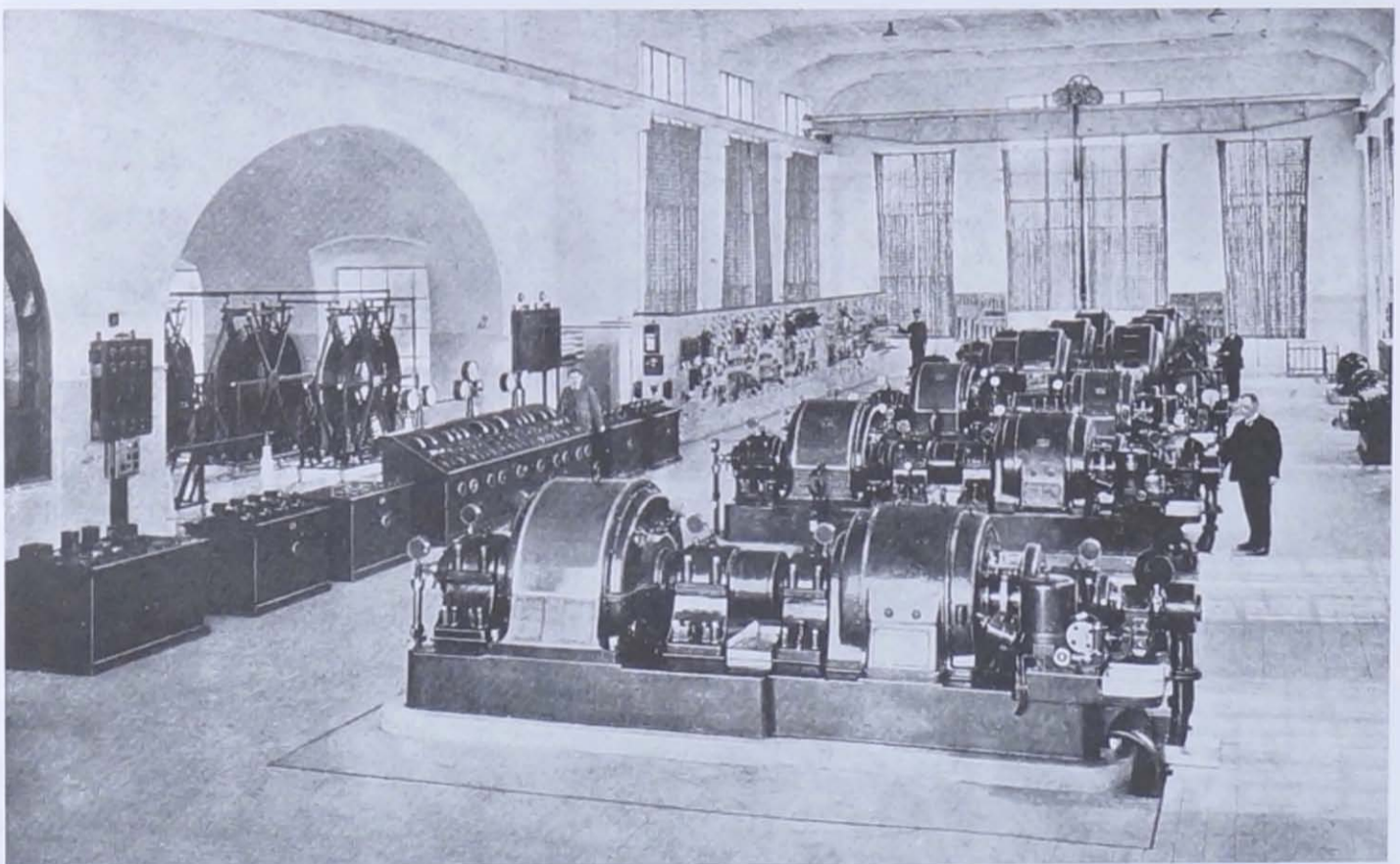
Machinezaal voor de lange golvenzender in Ruiselede omstreeks 1930. (3)
