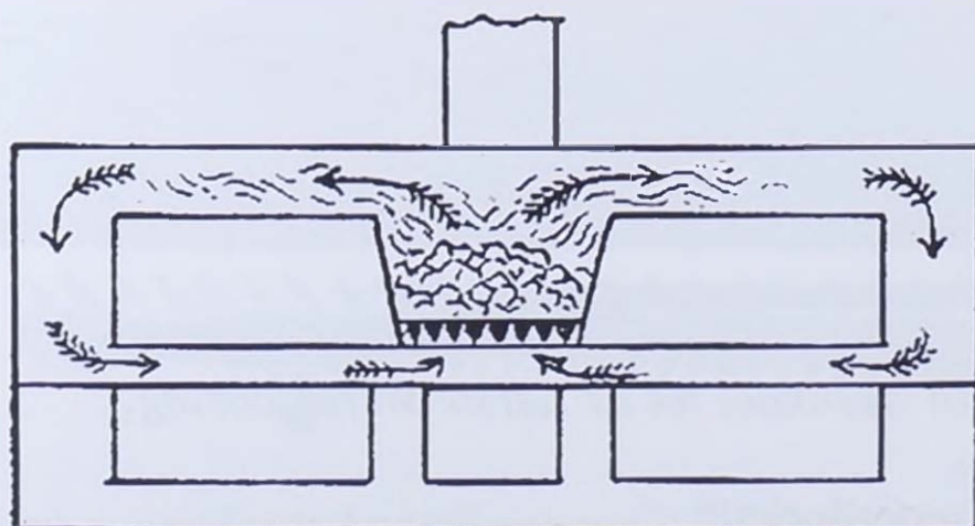
Principe van de luchtcirculatie in een cuisinière. (8)
