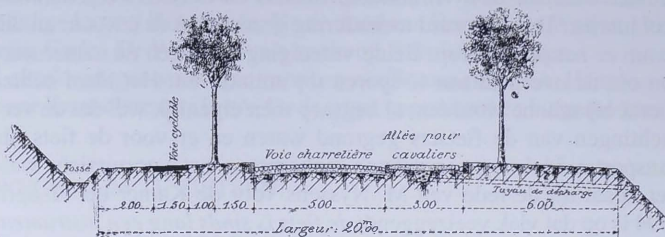
Modelprofiel voor de aanleg van grote wegen. (29)
