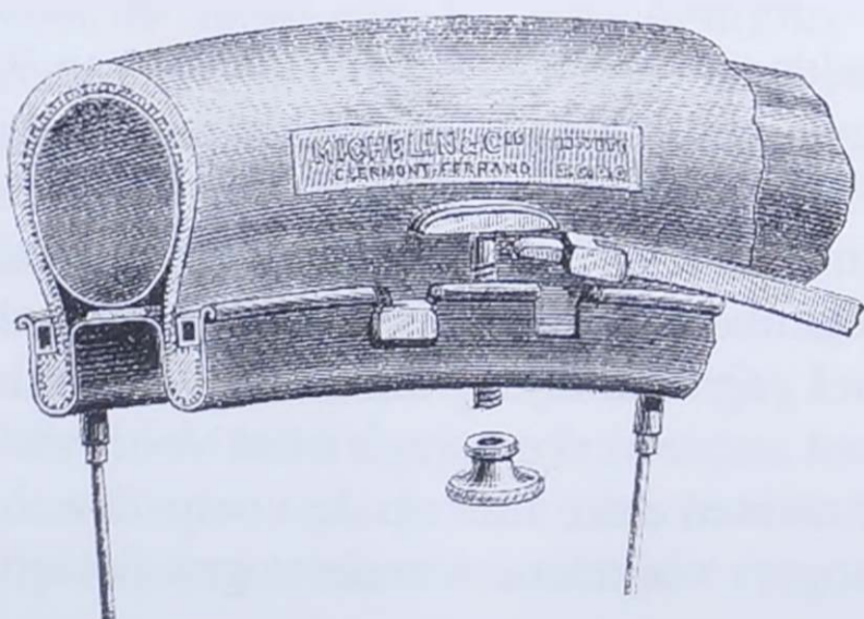
De eerste verwisselbare en herstelbare fietsband van Michelin anno 1897. (10)
