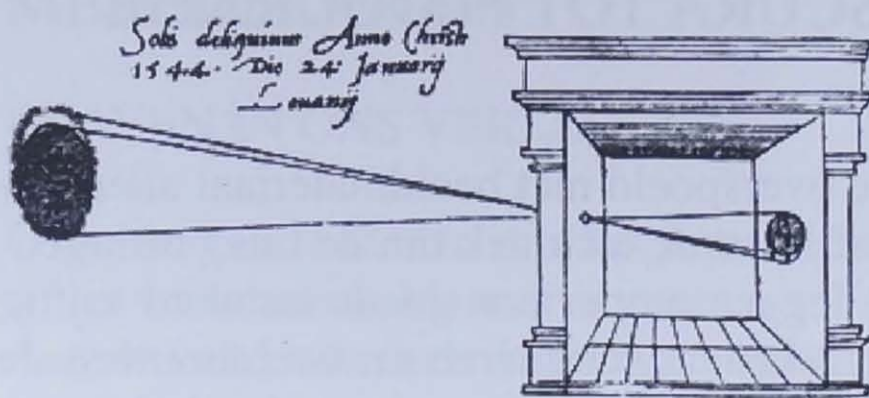
Observatie van de zonsverduistering van 24 januari 1544 door Gemma-Frisius.
