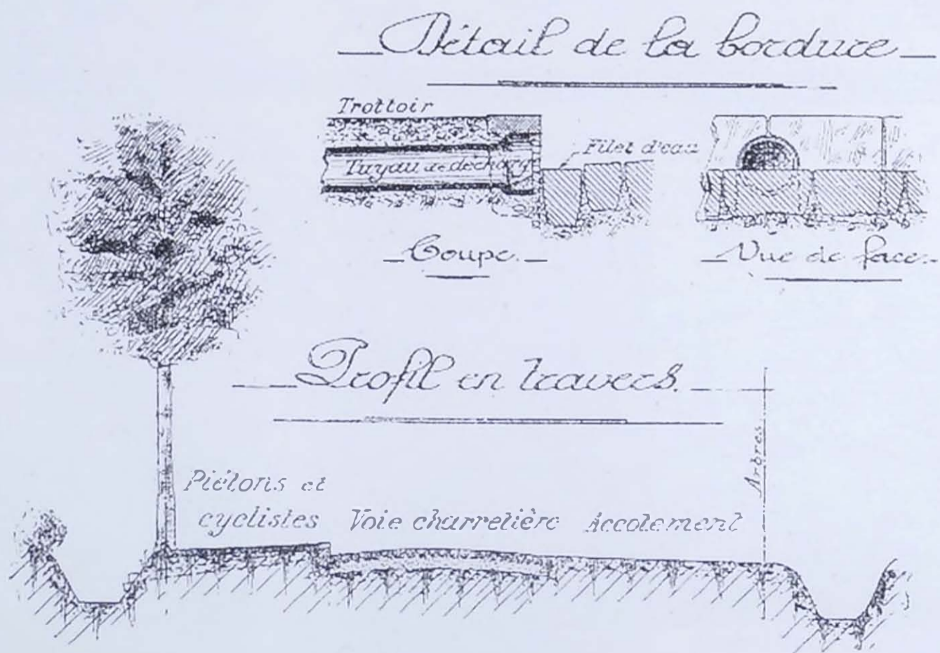
Model van wegprofiel bij de aanleg van fietspaden. (33)
