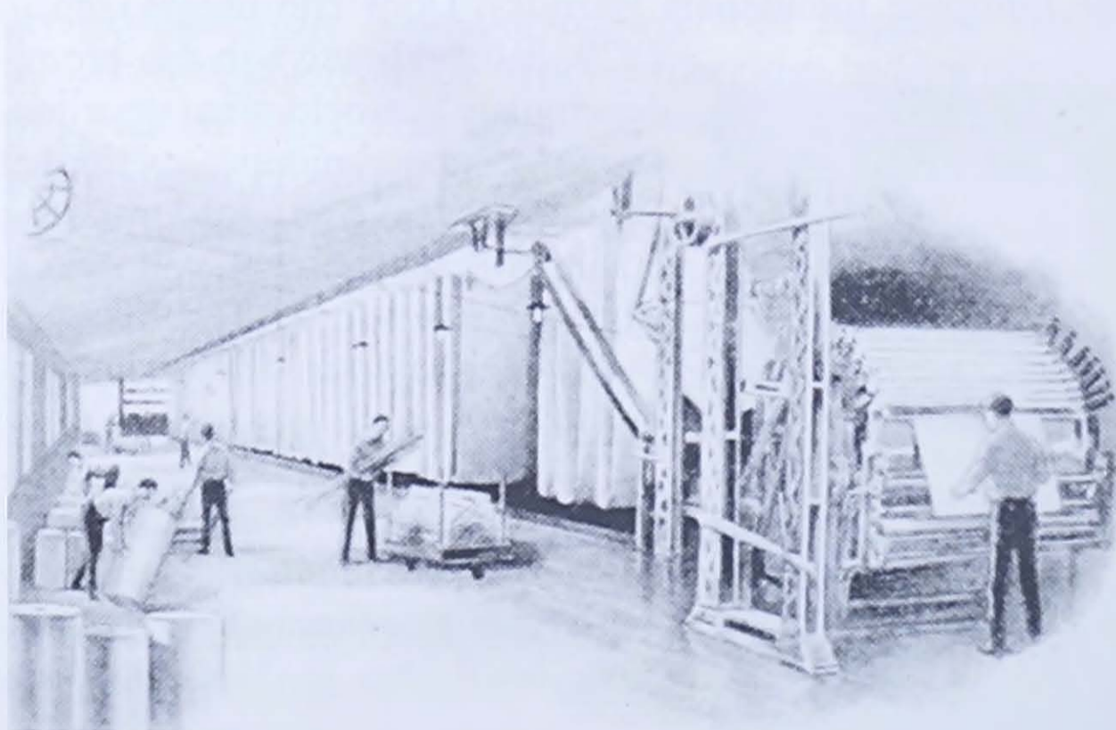
Zicht op een deel van de productieketen van het Velox-papier in het bedrijf van Baekeland.
