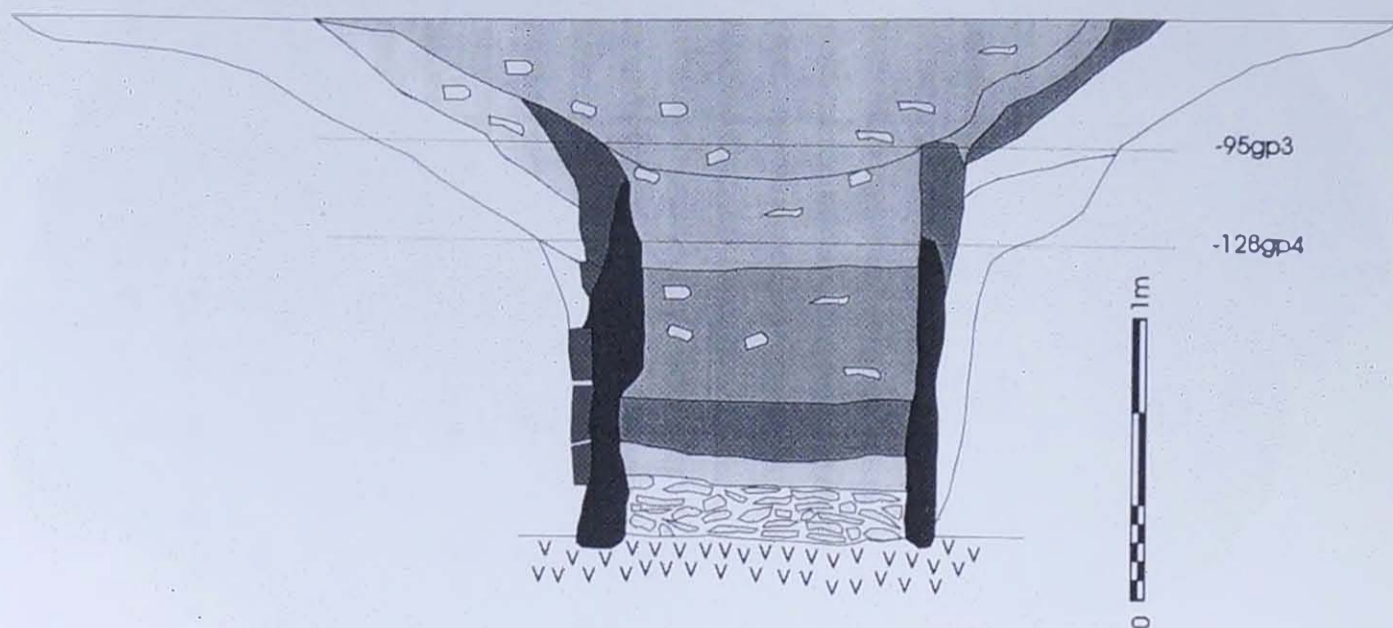
Doorsnede van een middeleeuwse waterput.
