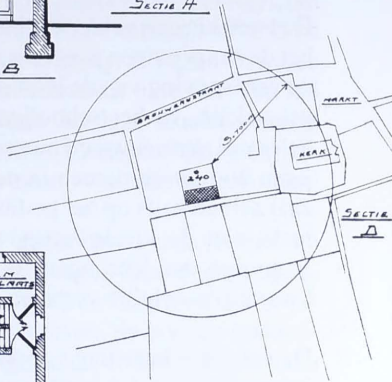
LIGGINGSPLAN - SCHAAL 1/2500
